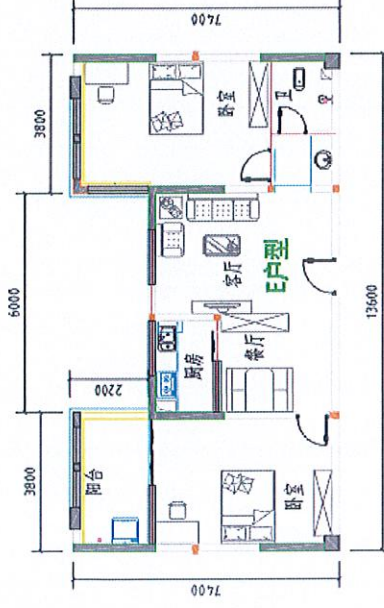
套内建筑面积E户型: 79.86㎡
