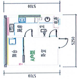
套内建筑面积A户型: 23.97㎡
