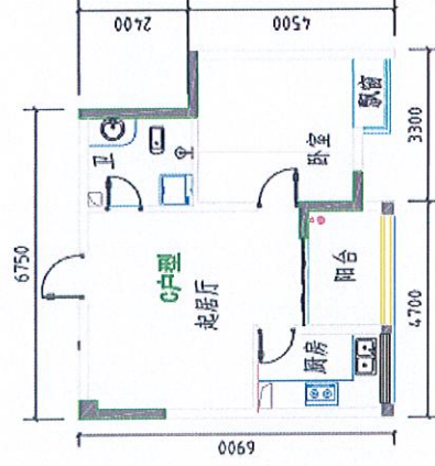
套内建筑面积C户型: 43.89㎡
