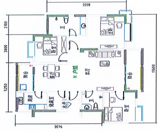
套内建筑面积H户型: 113.78㎡
