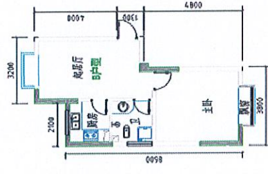
套内建筑面积B户型: 40.14㎡
